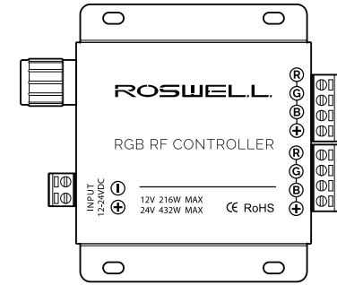
RGB Controller
